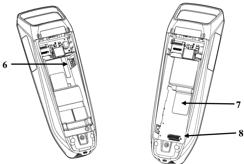
Рисунок 4 Внутреннее устройство РВ КМ
