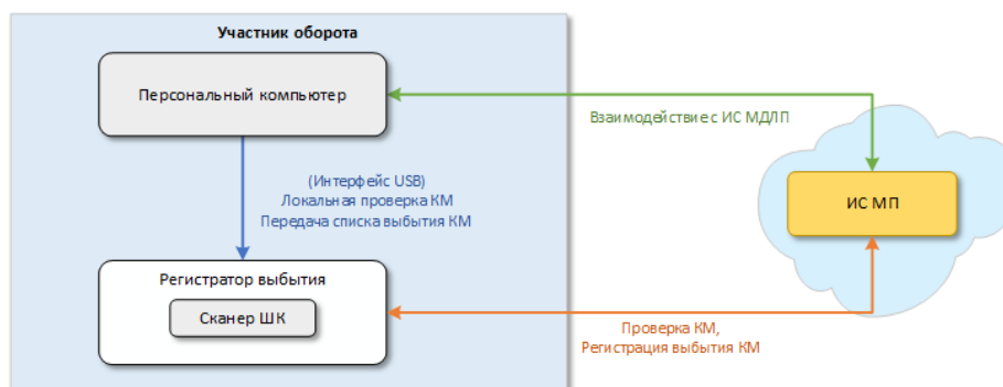
Рисунок 6 – Вариант локального подключения РВ КМ
